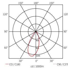
MCR-PL1 30K-24V-46-BK
